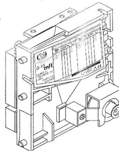
Рисунок 1 – Устройство монетоприемник монет номиналом 1 рубль, 3 рубля, 5 рублей, 10 рублей
